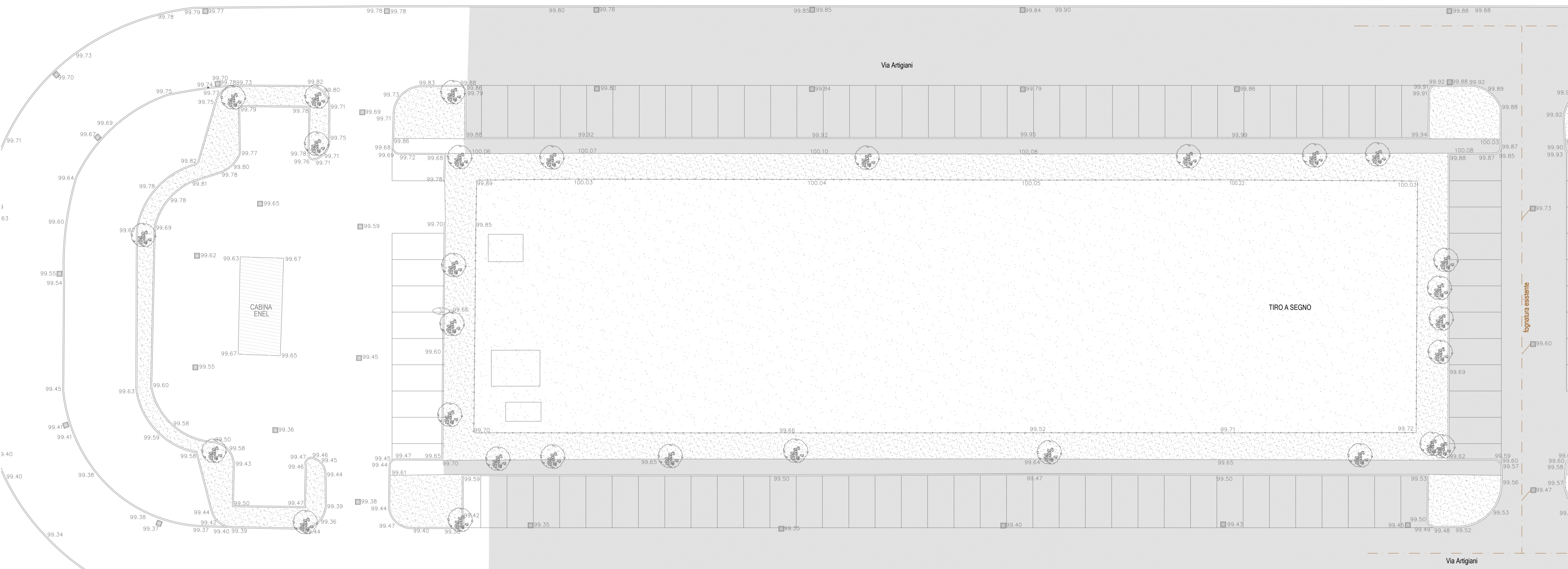
PLANIMETRIA GENERALE scala 1:200
